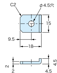
サーボマウント金具 (オプションのフランジに付属)
